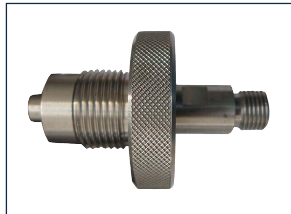
M26-1/4''-BU-300B-RVS-Conisch Bestelnummer: 120-00203
