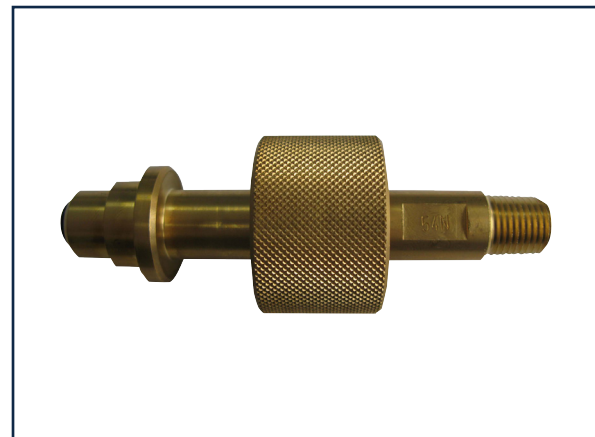
HI-Helium-CEN-300B-1/4-BU Bestelnummer: 120-00366
