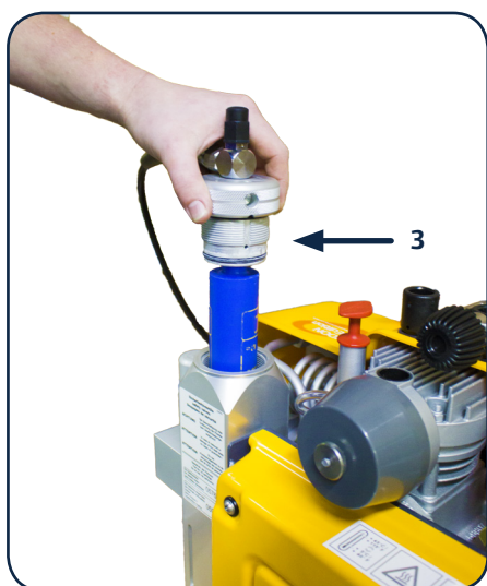
2. Haal het filterpatroon uit het filterhuis omhoog
