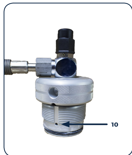
10. Komt er uit dit voorste gaatje lucht, dan zit het filterpatroon er niet goed in of de O-ringen van het filterpatroon zijn beschadigd
