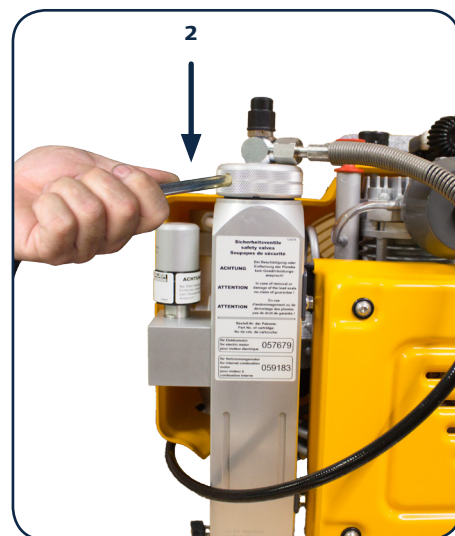
2. Draai de filterkop open tegen de klok in
