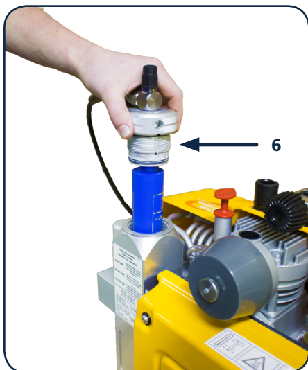
6. Plaats het filterpatroon terug in het filterhuis
