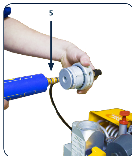
5. Plaats het filterpatroon in de filterkop, druk deze stevig aan, deze moet klikken
