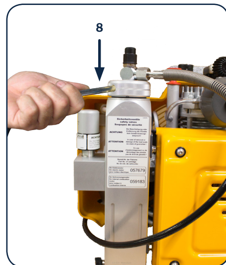
8. Draai de filterkop weer in het filterhuis met de klok mee tot deze compleet vast zit. Draai hem dan 1/8 slag weer tegen de klok in, dus heel iets losser. Nu is hij goed gemonteerd
