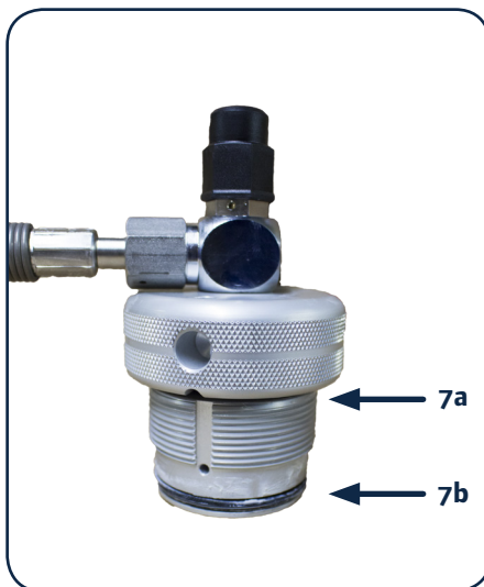
7a. Controleer de O-ring (115-00015), deze dient ter bescherming 7b. Controleer de O-ring (115-00039), deze is voor de afdichting
